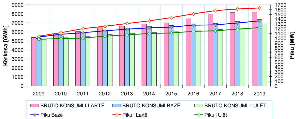
Fig. 3-6 Skenari i rritjes së ulët, mesatare dhe të lartë të bruto energjisë dhe piku i kërkesës
