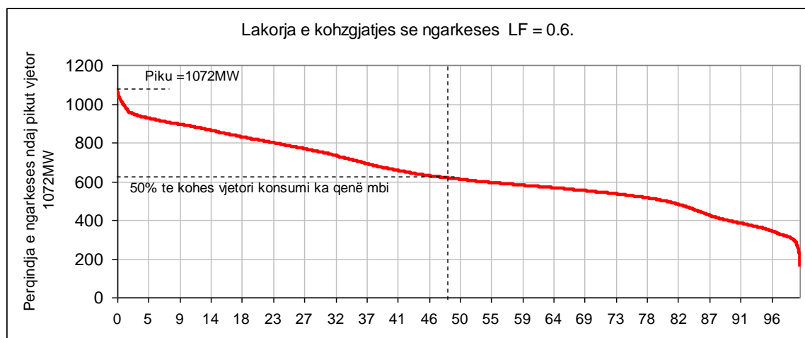
Fig. 3-3 Lakorja e kohëzgjatjes së ngarkesës për vitin 2009
