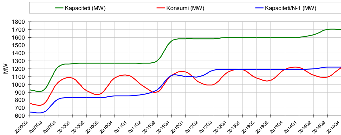
Fig. 6-8 Zhvillimi i kapaciteteve të rrjetit të transmisionit të planifikuara kundrejt konsumit nga 2009 deri në fund të vitit 2014
