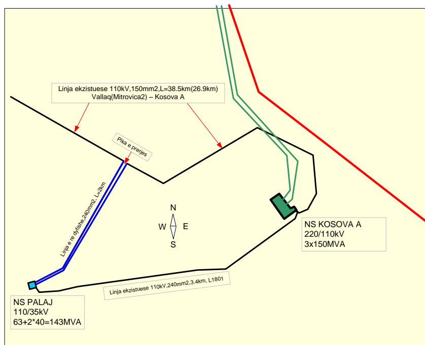
Fig.5-11. Projekti i përforsimit të kyçjes të NS Palaj
