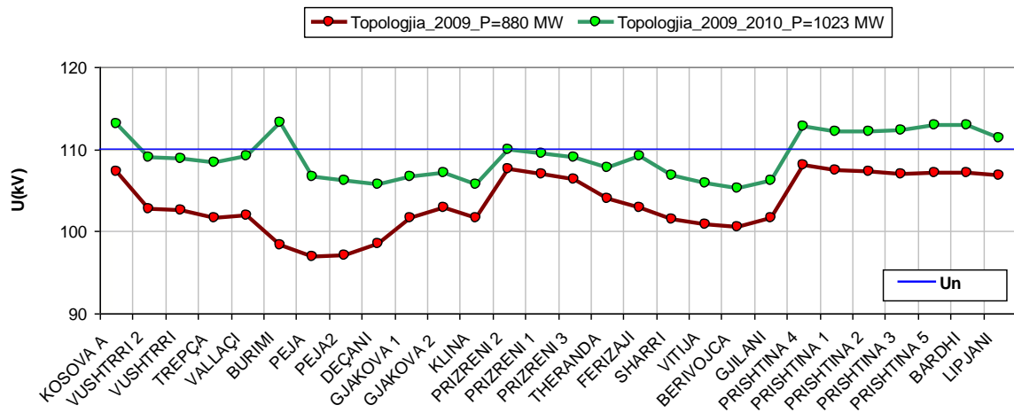
Fig. 6-3 Krahasimi i profilin të tensioneve para dhe pas përforcimeve në vitin 2009
