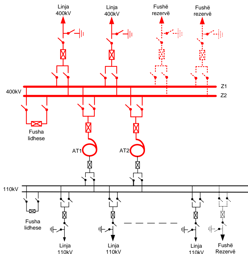
Figura 2-2 Planifikimi standard i konfiguracionit të zbarrave të nënstacioneve të reja të planifikuara në rrjetin e transmisionit
