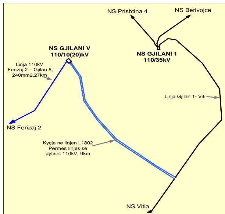
Fig.5-12. Projekti i NS Gjilani 5
