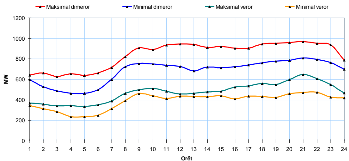
Fig. 3-5 Diagrami i zakonshëm ditor maksimal dimëror – veror dhe minimal dimëror- veror i zgjedhur në vitin 2009
