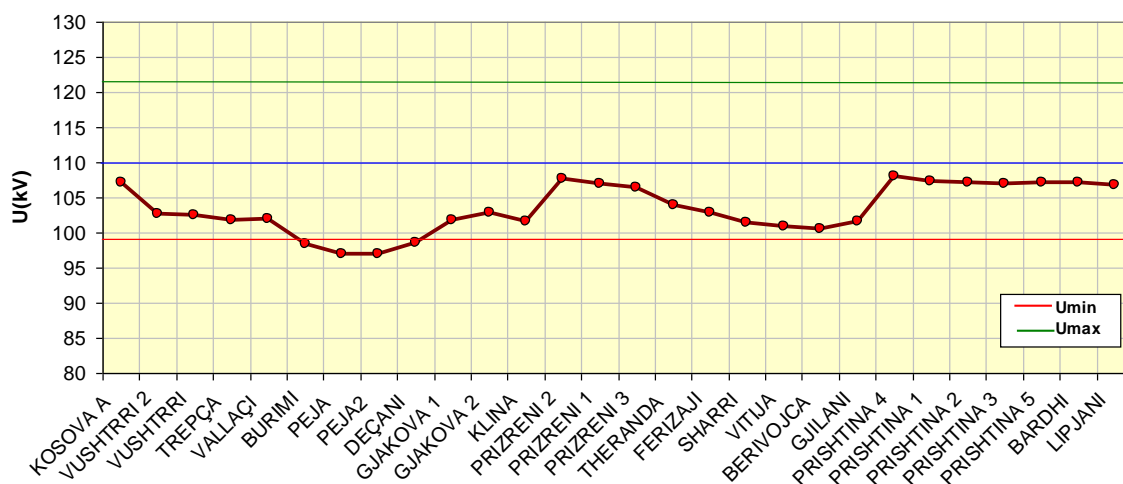
Fig 6-1. Profili i tensionit ne rrjetin 110 kV para futjes në operim të NS Peja 3 - për konsumin 880 MW
