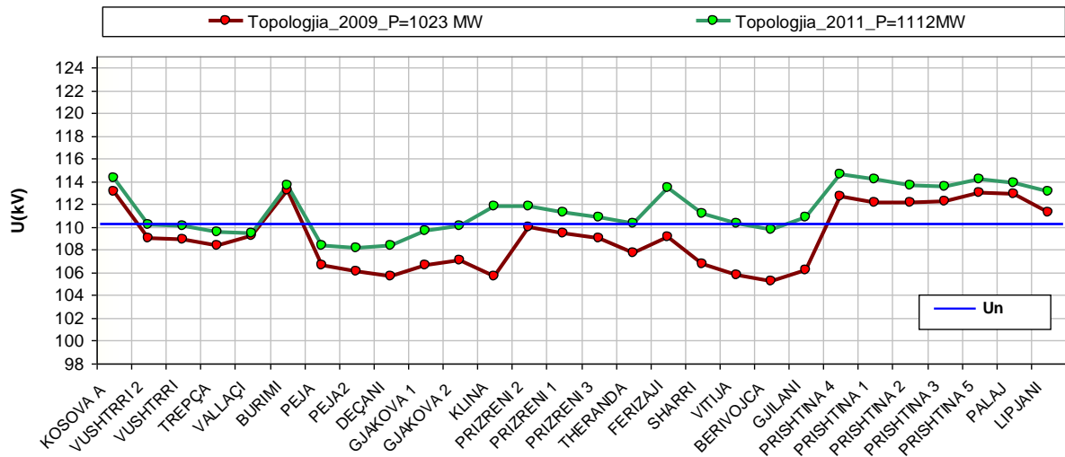
Fig. 6-5 Krahasimi i profilit te tensioneve 2009-2011
