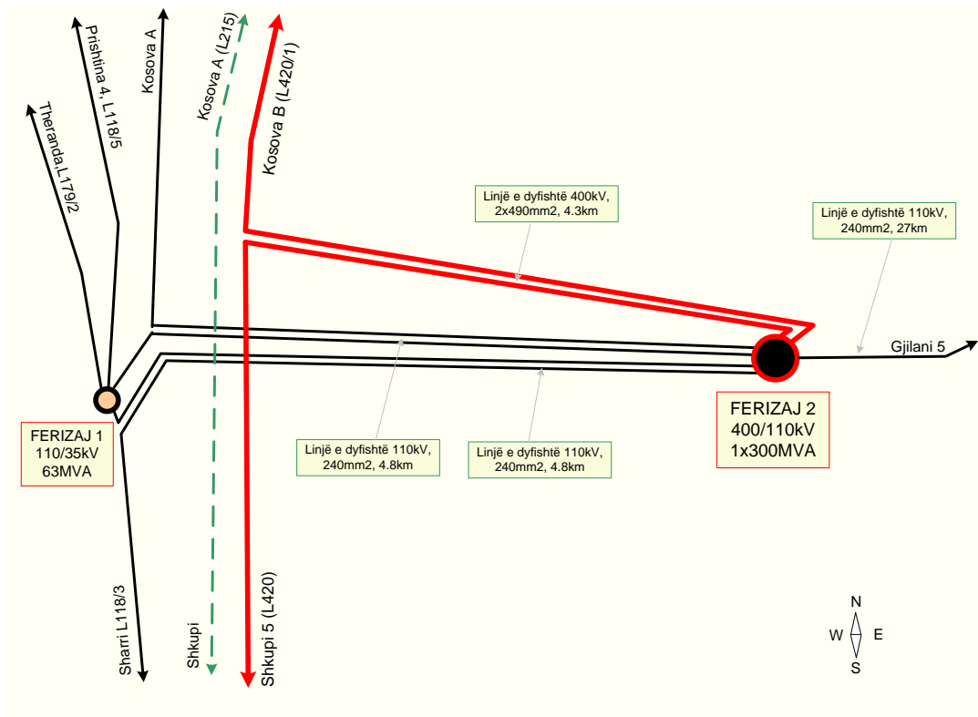
Fig.5-5. Paket Projektit Ferizaj 2, 400/110 kV ndërlidhja e tij në rrjetin e transmisionit
