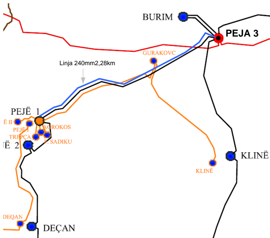
fig.5-10 Shtrirja gjeografike e linjës së re 110 kV NS Peja 3 – NS Peja 1
