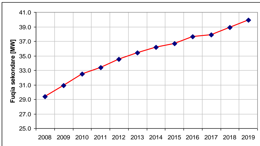
Fig.5-14 Parashikimi i nevojave të fuqisë rregulluese sekondare
